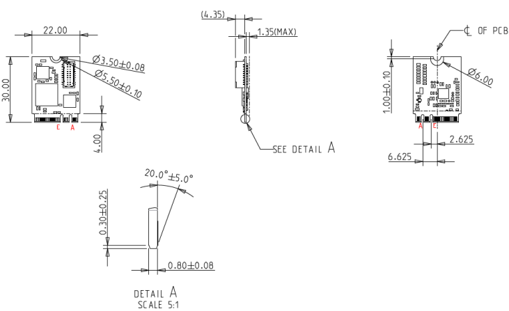
EGP2-X201-W1 (Vertical Connector)
