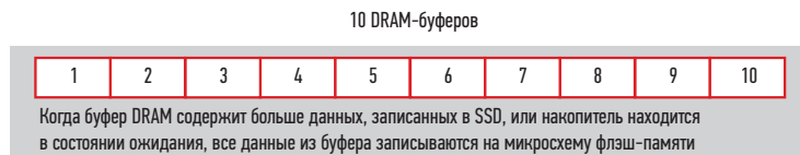
РИС. 3. ◀ Применение iCell Technology с накопителями 3MG2-P/3MR2-P/3SR3-P/3SE2-P
